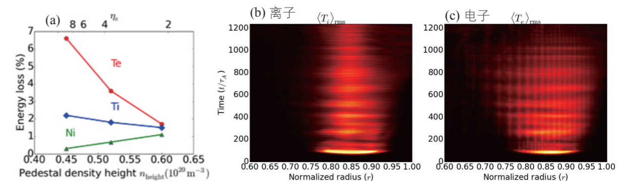
图 1: (a) 随着台阶区密度升高，电子温度提供的能量损失显著降低，与实验相符；(b) 离子湍流的径向宽度随着时间没有变化，没有湍流径向传播效应；(c) 由于湍流径向传播效应，电子湍流的径向宽度随着时间逐渐增加，图中的竖条纹是由电子朗道阻尼效应产生的。
