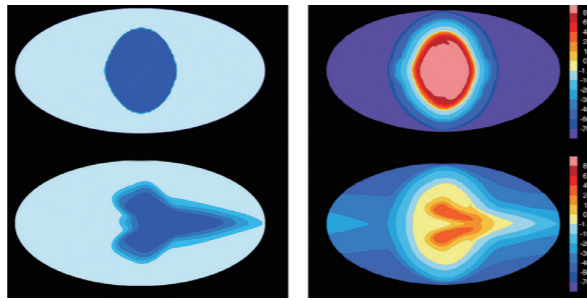
图：气候模式模拟的海冰覆盖率（左）和温度分布（右）。上图：静止的海洋。下图：动态海洋。左图中的蓝色表示开放海域，白色表示冰封海域。右图的彩色标尺单位是 ^{\circ}\text{C} 。恒星的直射点在图的中心。
