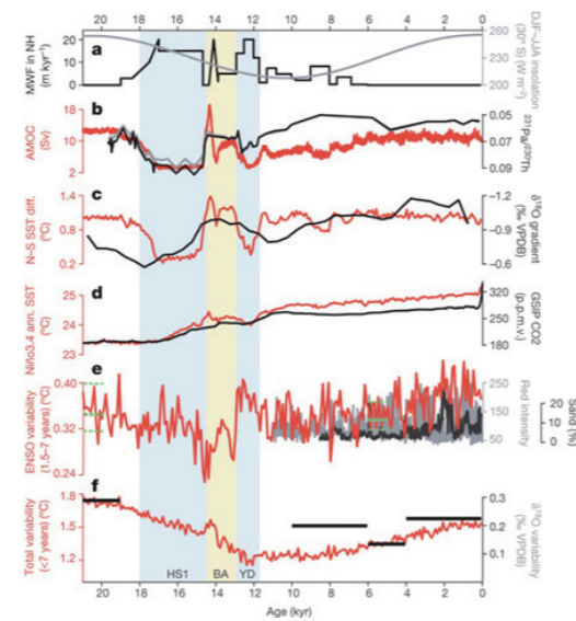
图 1：21000 年来主要气候强迫的变化和厄尔尼诺的响应。a) 北大西洋淡水通量（黑线）与南纬 30 度冬-夏太阳入射能量的差异（灰线）；b) 北大西洋经向翻转流（红线）与百慕大地区 231Pa/230Th 比值（黑、灰线）；c) 东太平洋经向海温差（红线）与氧同位素记录（黑线）；d) Nino3.4 区的海温指数（红线）与 CO2 重建序列（黑线）；e) 厄尔尼诺年际振幅（红线）以及东太平洋（黑线）和南美沿岸（灰线）的湖泊沉积记录，绿线是 PMIP 计划模拟结果的范围；f) Nino3 区海温 7 年以下的总变率，黑线是东太平洋沉积记录的总变率。
