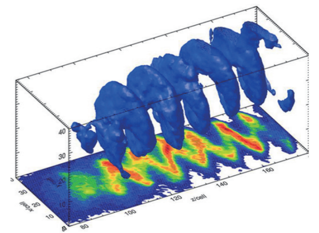
图 1 电子束能量密度三维分布图 Fig.1 Energy distribution of electron beam in 3D space
