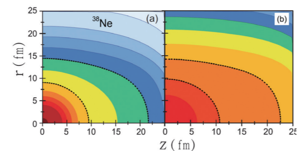
图 1: 坐标空间 HFB 计算首次预言出 ^{38}\text{Ne} 可能有蛋形晕结构 (中心部分为球形, 外部为形变晕)。(a), (b) 分别为中子晕与中子对密度晕。
