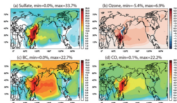
图1: 2006年中国产品出口的相关污染物及前体物排放对北半球近地面大气中的污染物浓度的百分比贡献:(a)硫酸盐颗粒物,(b)臭氧,(c)碳颗粒物,(d)一氧化碳。
