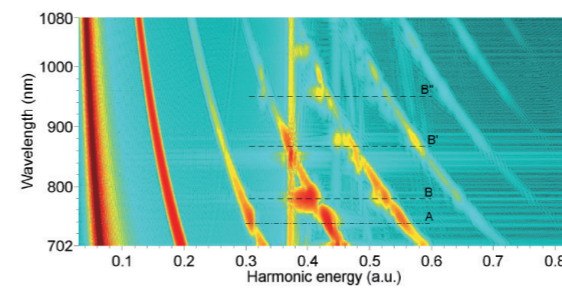
图 2: 氢原子不同激光波长下的谐波辐射信号, 激光强度为 6 \times 10^{12} W/cm 2 。从图中可以看出随着波长变化, 谐波产率受到很大的调制, 出现很多共振峰和原子线跃迁辐射。
