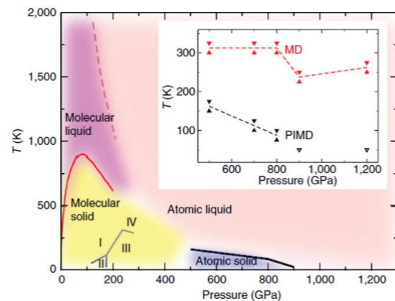
图 1: 高压下的氢相图，以及经典（量子）统计下固体氢的融化曲线。
