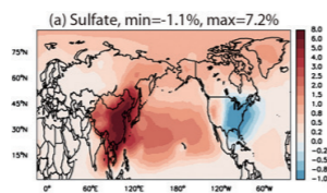
图2a: 2006年美国从中国进口产品与自身生产相应产品相比,对北半球近地面大气中的硫酸盐颗粒物浓度的百分比影响。
