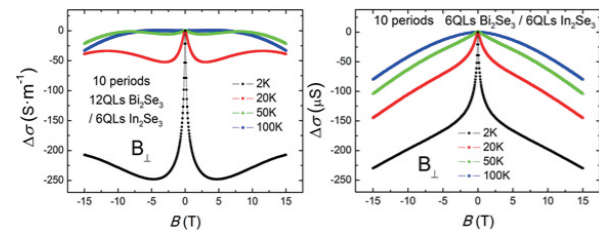
图：(Bi2Se3)12/(In2Se3)6 和 (Bi2Se3)6/(In2Se3)6 超晶格的量子输运特性
